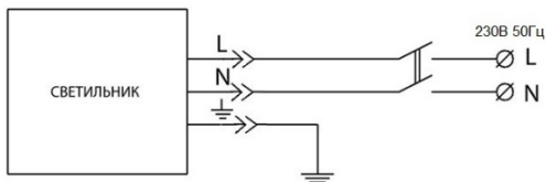
Рисунок 3 Схема подключения светильника
