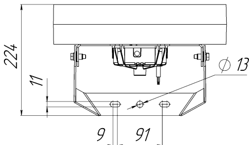
Рисунок 2. Светильник Wheel с кронштейном
